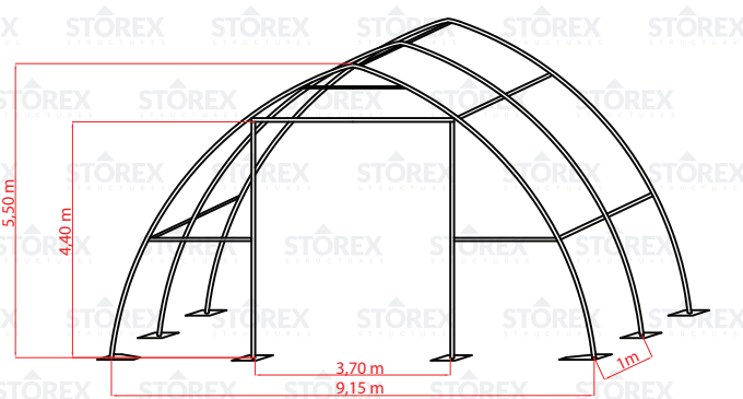
Dibujo dimensional parcial (no se muestran todos los arcos de marco)
