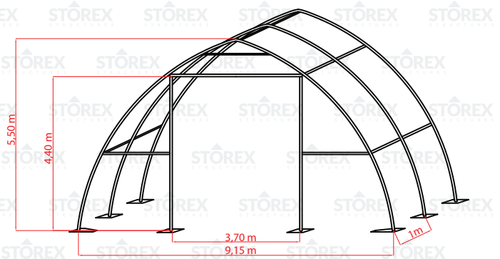
Dibujo dimensional parcial (no se muestran todos los arcos de marco)
